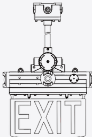
Pendant Mount
